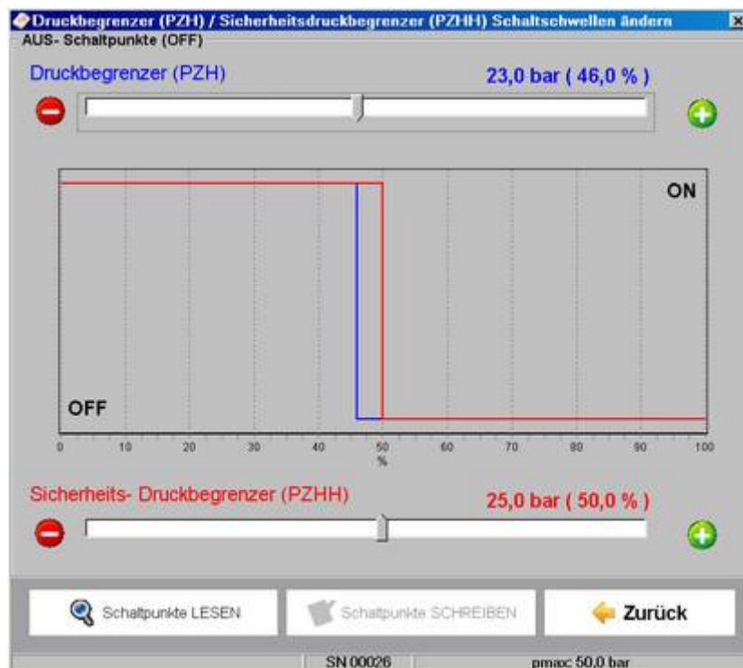
Fig. 6: Einstellung Schaltschwellen (Version 2.0)
